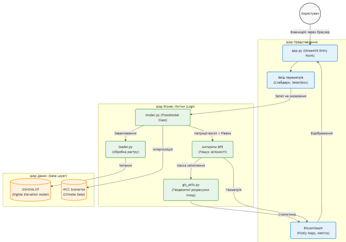
Рисунок 2.1 – схема архітектури програмної частини [26]
